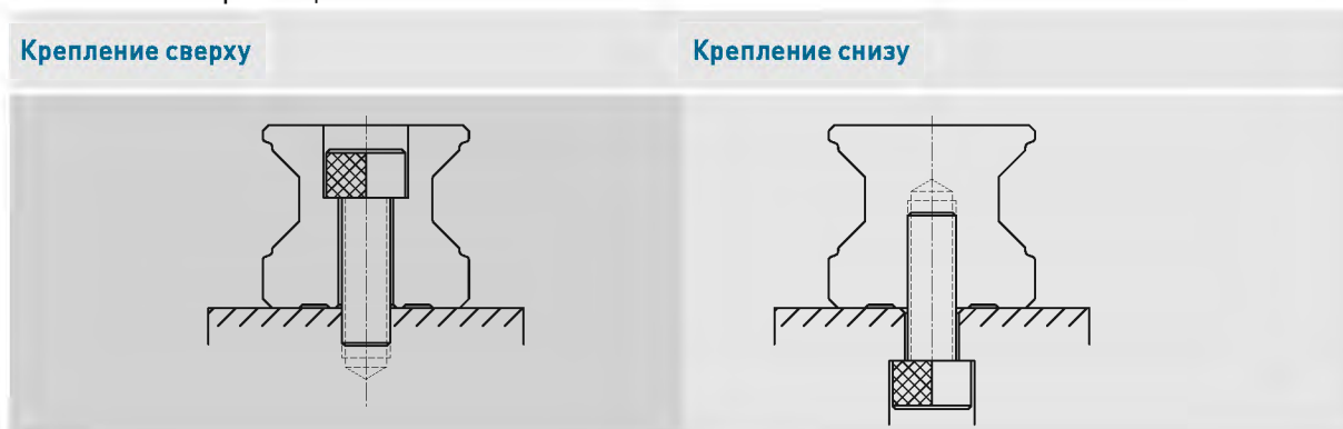
Табл. 2-7-3 Типы направляющих
